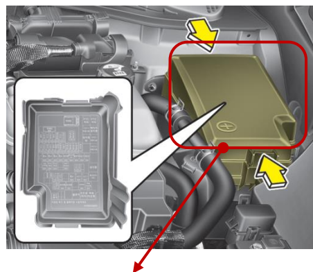
Scatola fusibili del vano motore
